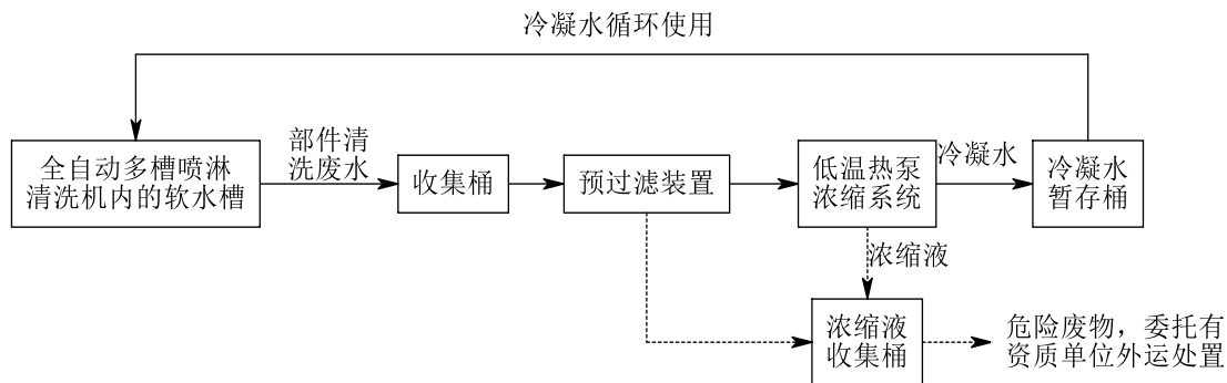
图 3-3 现有部件清洗废水处理设施处理工艺示意图
