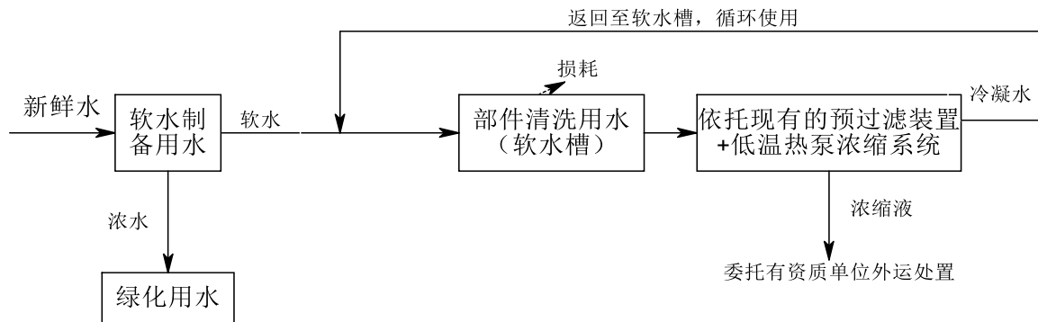
图 3-2 本项目废水处理流程示意图
