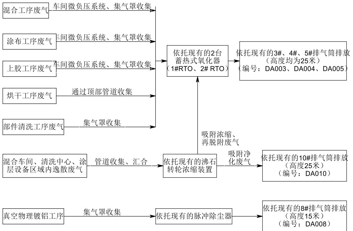
图 3-1 本项目废气处理流程示意图
